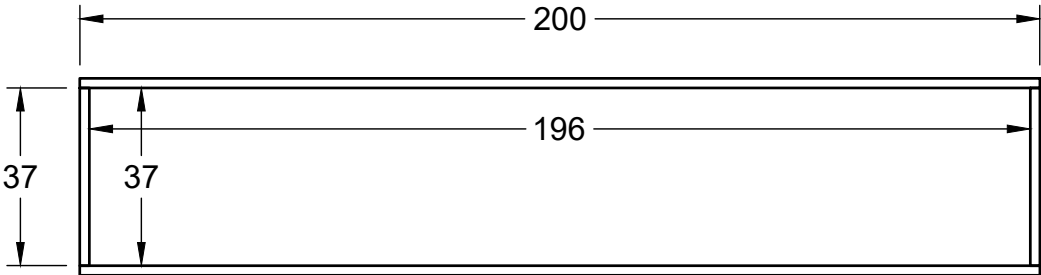
Top
